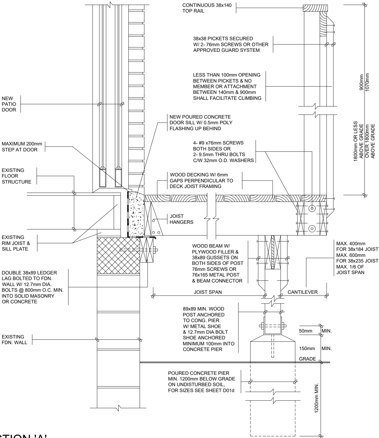
SECTION 'A'
