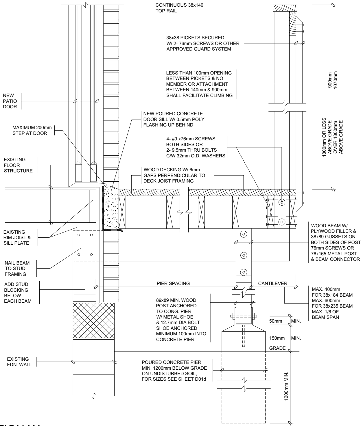
SECTION 'A'
