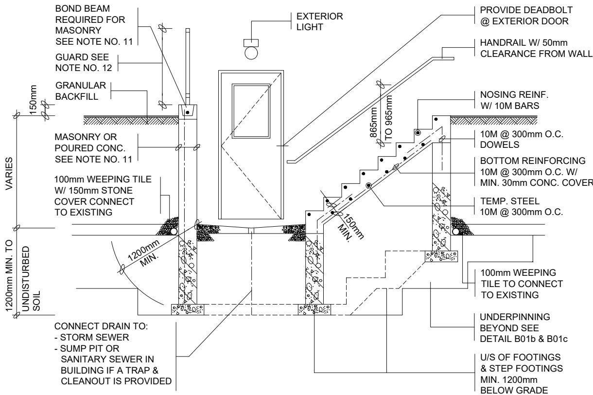
SECTION 'A'
